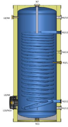
ÇİFT SIRA SERPANTİNLİ ISI POMPASI BOYLERİ
