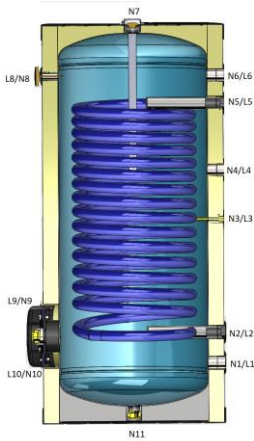
TEK SIRA SERPANTİNLİ ISI POMPASI BOYLERİ
